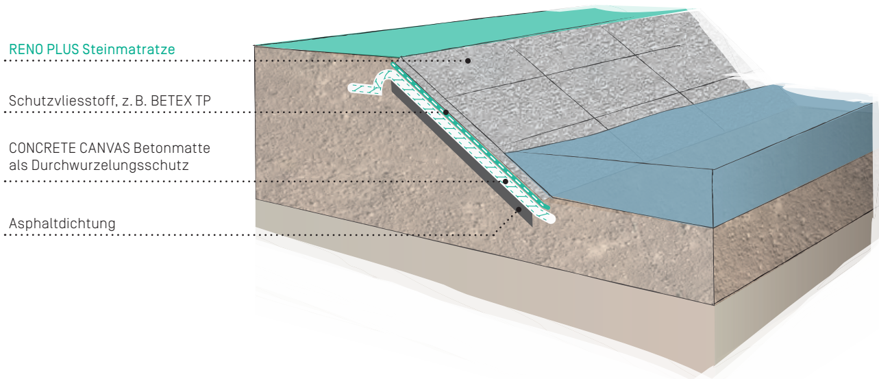
Ufersicherungssystem auf bestehender Dichtung
