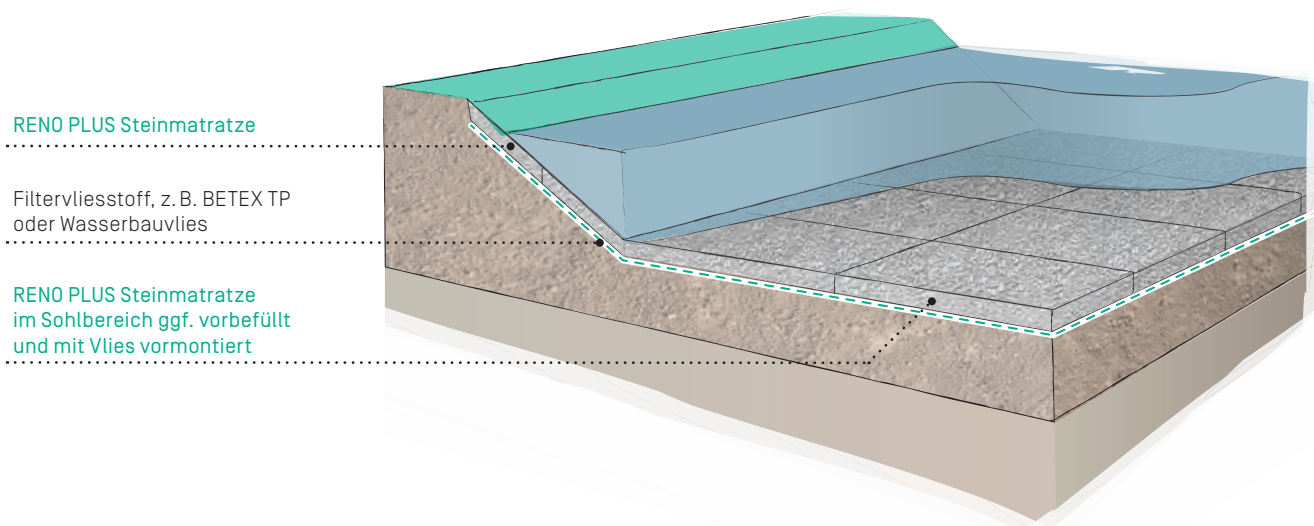
Uferböschungssicherung und Sohlsicherung z. B. gegen Schraubenverwirbelung
