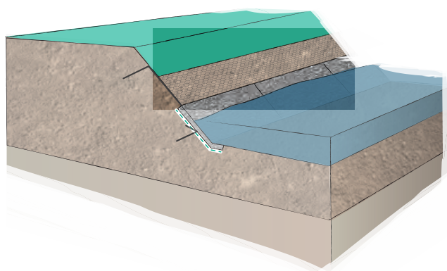
Aufgehängtes Deckwerk
